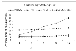
Fig. 22. Query evaluation time w.r.t. k .
